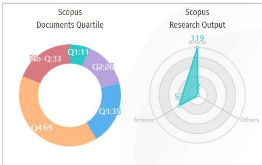
Gambar 3 Data Publikasi pada Scopus Universitas Islam Negeri Raden Fatah Palembang
