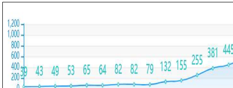
Gambar 1 Diagram Jumlah Publikasi Universitas Islam Negeri Raden Fatah Palembang.
