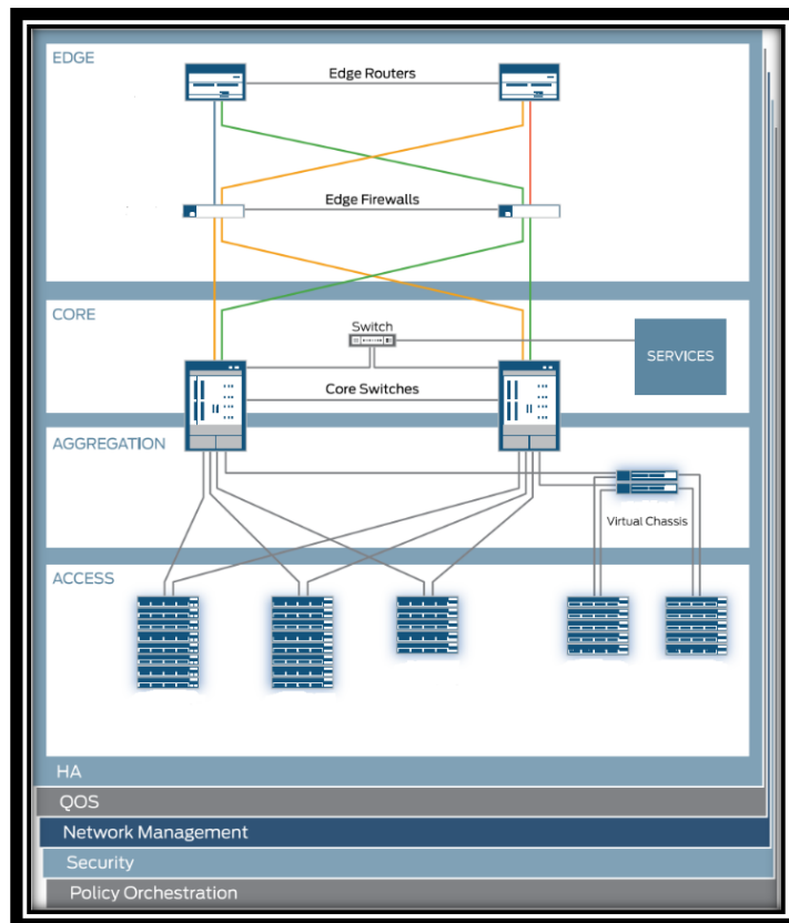
Gambar 7. Contoh Solusi Arsitektur Midsize Enterprise Kampus
